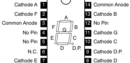
NTE3052, NTE3053 NTE3054, NTE3055
