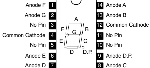
NTE3056, NTE3058 NTE3059, NTE3060
