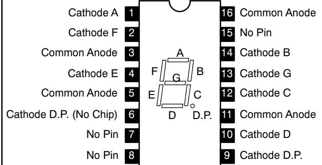
NTE3080, NTE3080-G, NTE3080-Y
